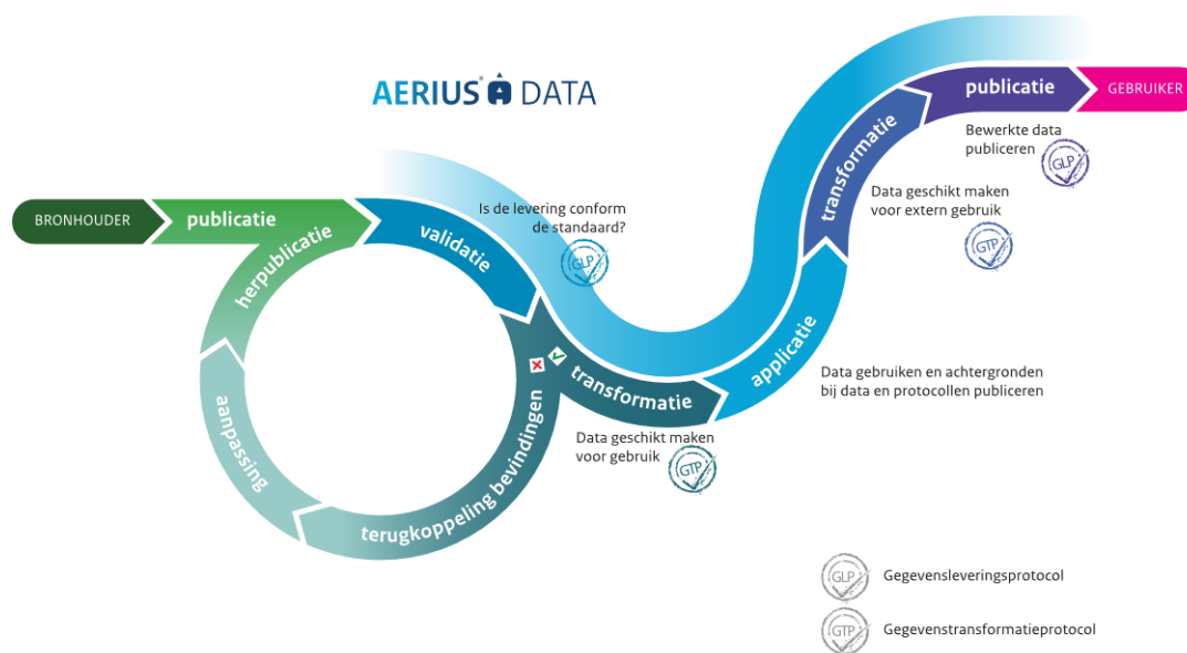
Figuur 38. Stroomschema gegevensbeheer in AERIUS
