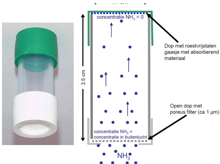
Figuur 4. Een Gradco-meetbuisje, ook wel passieve sampler genoemd. Deze metingen worden samen met het LML gebruikt om maandgemiddelde ammoniakconcentraties te verkrijgen. Bron: https://www.rivm.nl/stikstof/meetnetten
