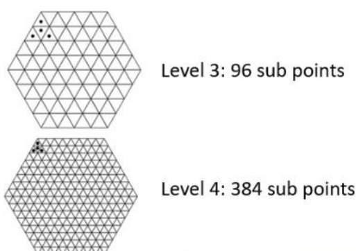
Figuur 8. Subreceptoren zijn zo verdeeld over het hexagoon, dat aan iedere subreceptor een even groot oppervlak kan worden toegekend (gelijke vlakverdeling).
