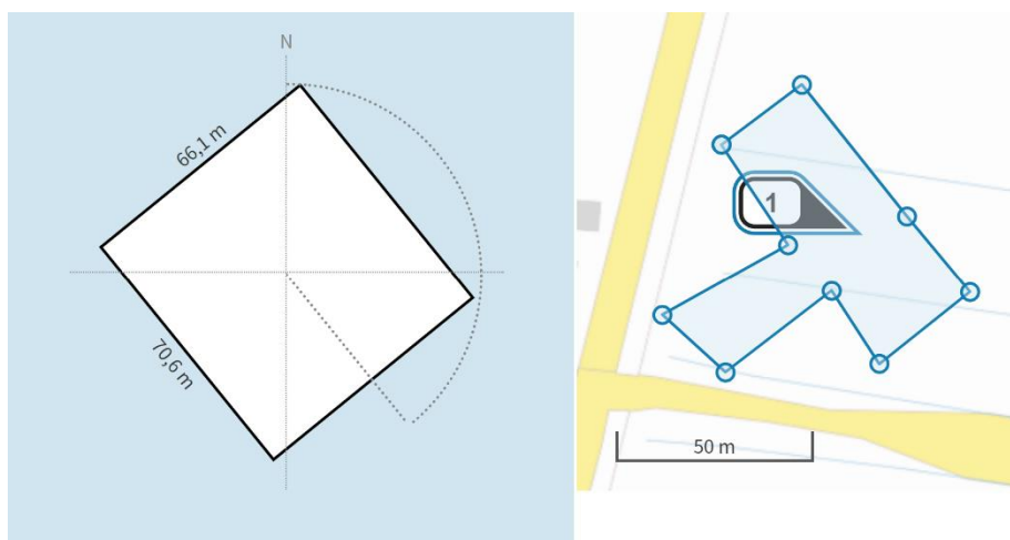
Figuur 17. Weergave van de envelop van een gebouw in AERIUS Calculator. De ingevoerde contouren (rechts) worden in de OPS berekening geïnterpreteerd als een rechthoekig gebouw (envelop) (links).
