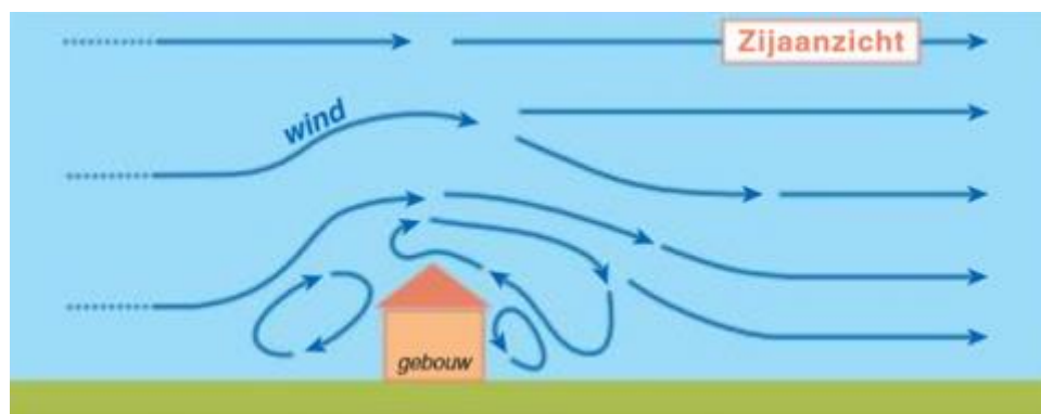
Figuur 14. Vereenvoudigde weergave van het effect van een gebouw op het windveld. Rondom het gebouw ontstaat (versterkte) turbulente werveling.
