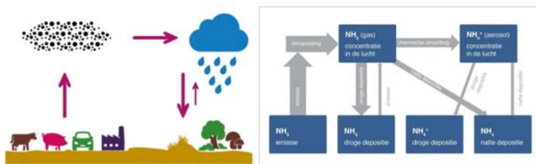
Figuur 5. Schematisch overzicht van de belangrijkste processen die een rol spelen in de luchtkwaliteit; links algemeen en rechts in detail geïllustreerd aan de hand van ammoniak. In het rechterdeel van de figuur zijn de fysische grootheden zoals concentratie en depositieflux vermeld in de blauwe blokken en geven de grijze pijlen de processen weer. De dikte van de pijlen is een (ruwe) maat voor het belang van het proces in de ammoniakketen; voor andere componenten kunnen de verhoudingen anders liggen.
