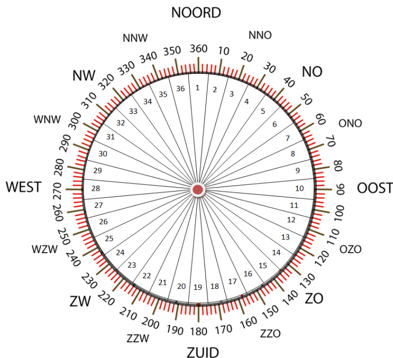
Figuur 43. De mogelijk voorkomende windrichtingen zijn ingedeeld in 36 windsectoren. LET OP: de oriëntatie van de windrichting in graden. Een windrichting van 0 graden komt overeen met noordenwind. Windrichting van 90 graden komt overeen met oostenwind.
