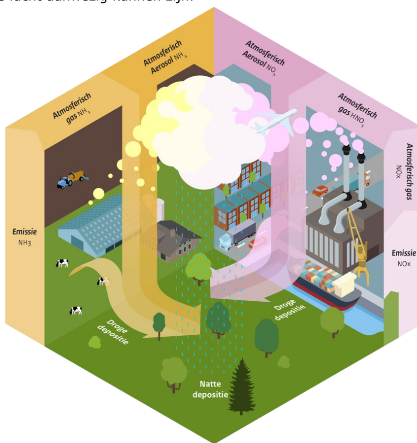
Figuur 2: Schematisch overzicht van het transport van stikstof door de lucht en de natte en droge depositie ervan. (Bron: Rijksinstituut voor Volksgezondheid en Milieu (RIVM), Ontwikkelingen in de stikstofdepositie, 2018)
