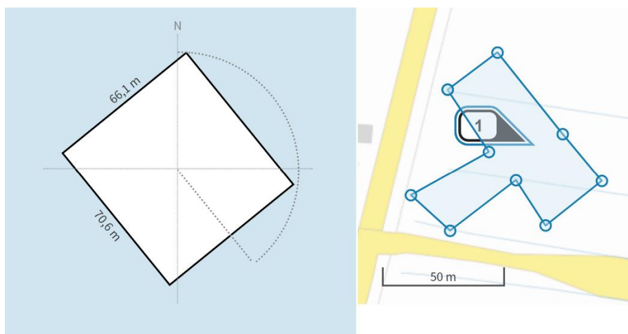
Figuur 27. Weergave van de envelop van een gebouw in AERIUS Calculator. De ingevoerde contouren worden geïnterpreteerd als de envelop (links) rondom het door de gebruiker getekende polygoon (rechts).
